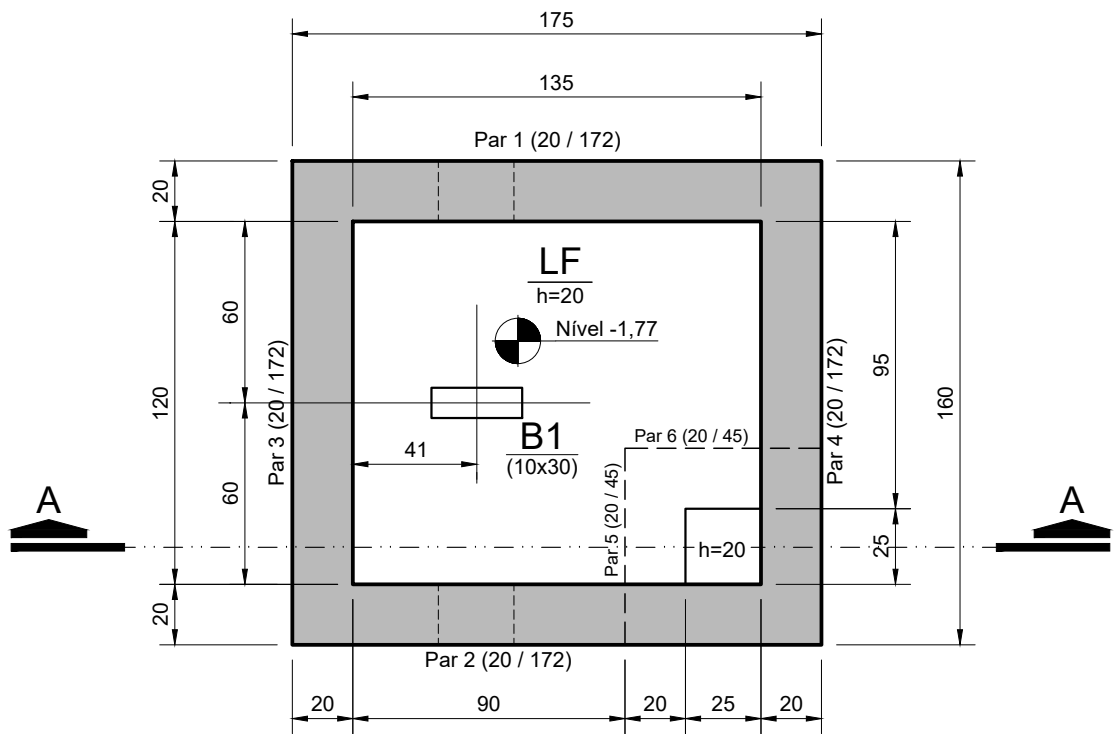
PLANTA BAIXA - Nível -1,77 escala 1:25
