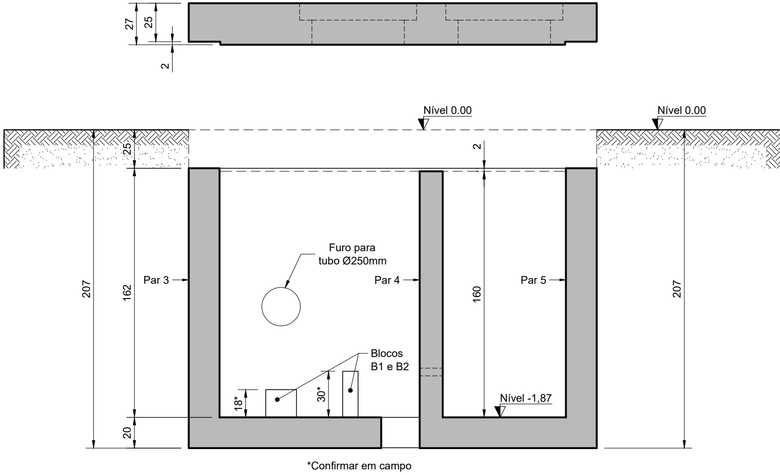
CORTE A-A
