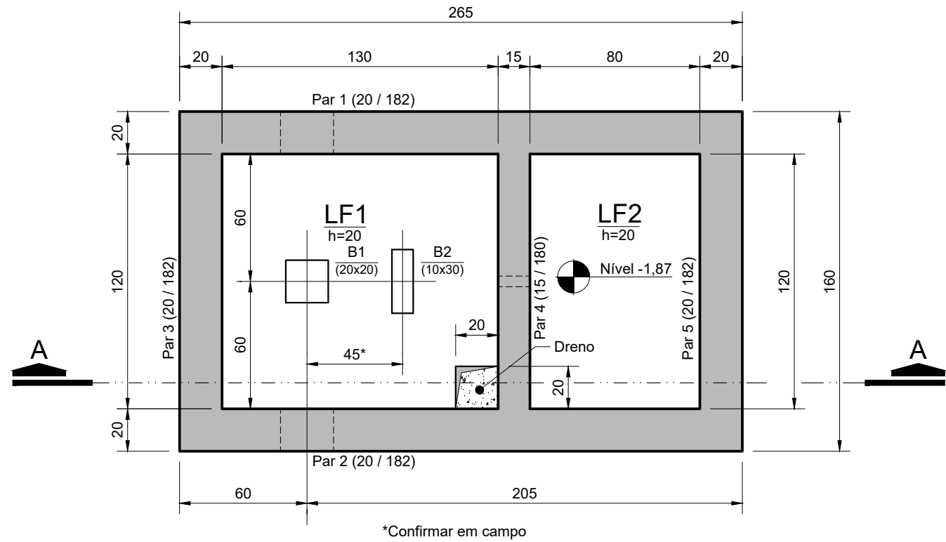
FORMA DA LAJE DE FUNDO - Nível -1,87
