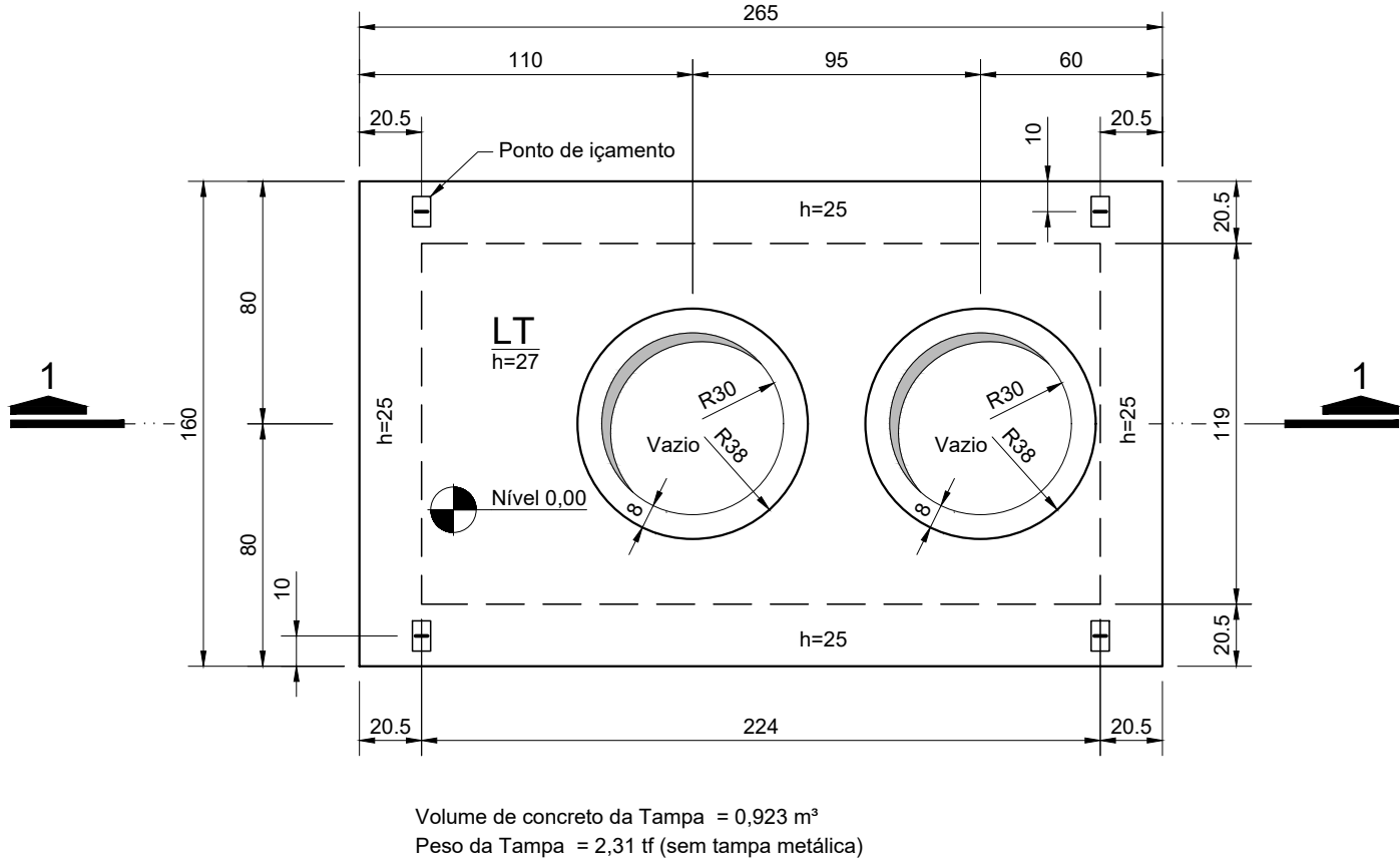
FORMA DA LAJE DE TAMPA - Nível 0,00
